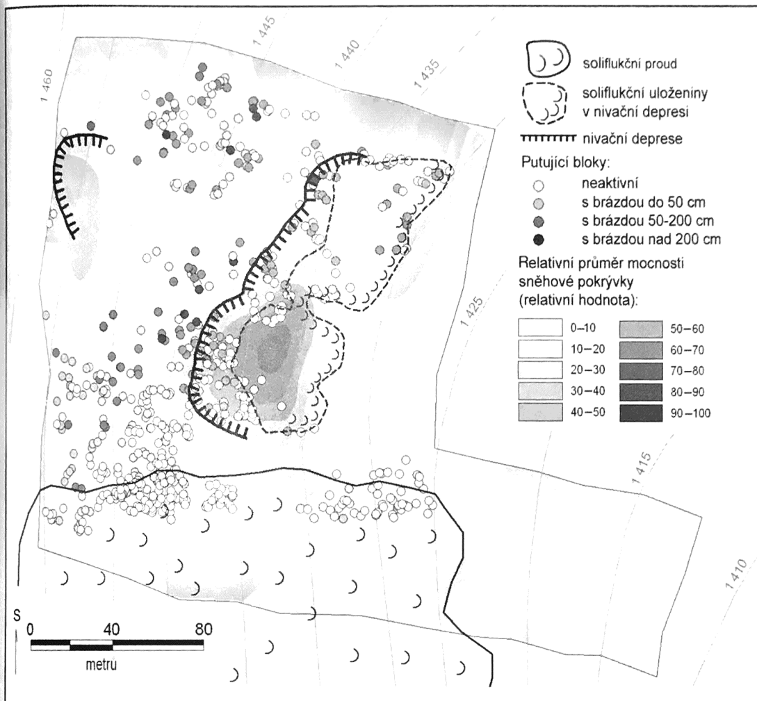
Obr. 4 – Relativní průměr výšek sněhové pokrývky a geomorfologie v lokalitě Čertovo návrší, období 2004–5. Relativní průměr je průměrem z map výšky sněhové pokrývky za každé měření přepočtených na relativní hodnotu 0 až 100 (viz metodika).
