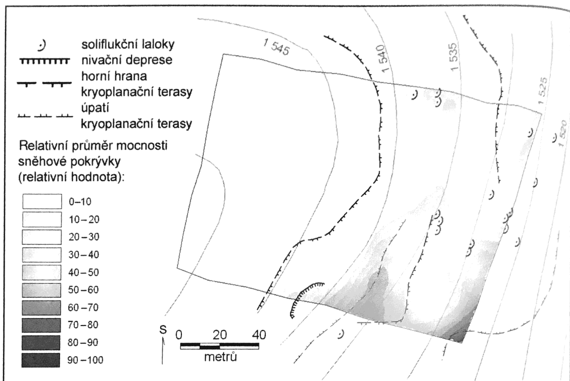
Obr. 7 – Relativní průměr sněžové pokrývky a geomorfologie v lokalitě Studniční hora, období 2004–5
