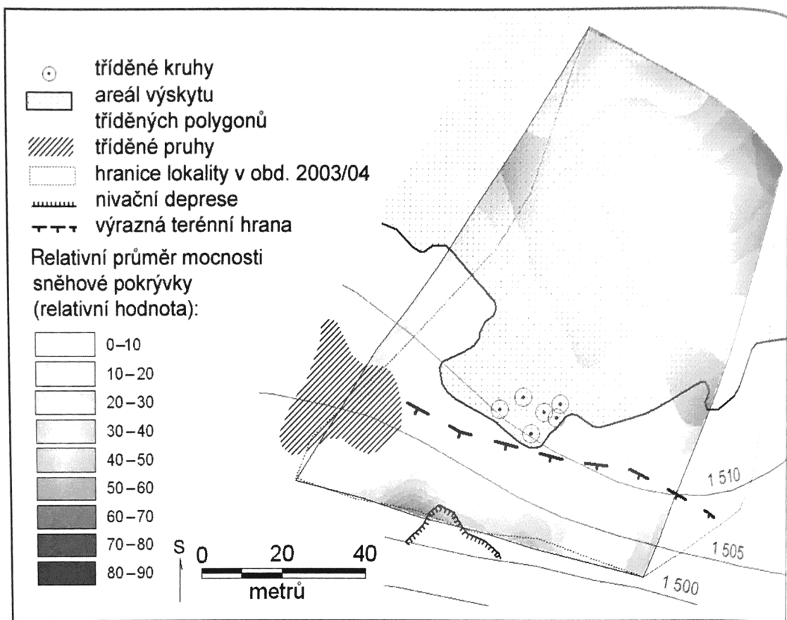
Obr. 10 – Relativní průměr sněhové pokrývky a geomorfologie v lokalitě Modré sedlo, období 2004–5
