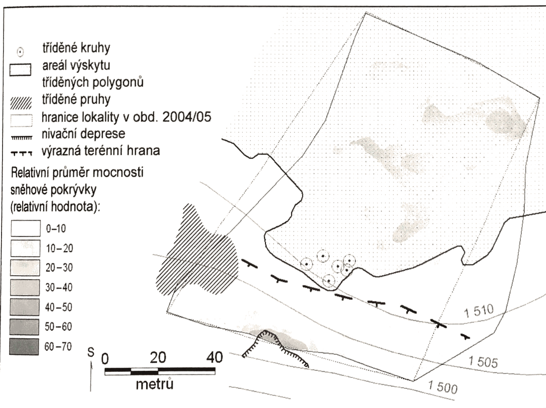
Obr. 9 – Relativní průměr sněhové pokrývky a geomorfologie v lokalitě Modré sedlo, období 2003–4
